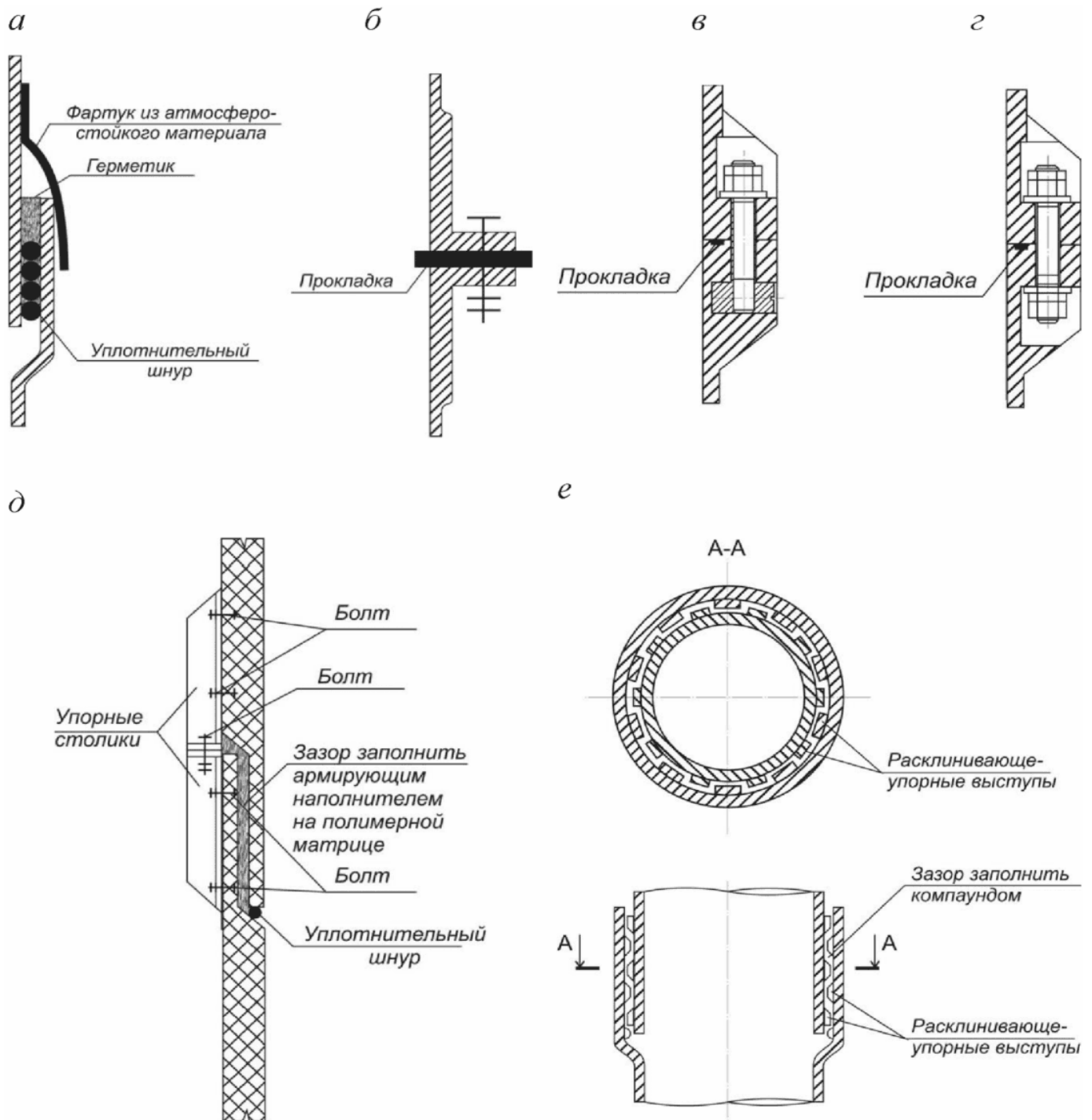
Рисунок 14.2 - Основные схемы соединений царг газоотводящего ствола: раструбное компенсационное (а), фланцевое (б), фланцевое штифтовое (в), фланцевое шпилечное (г), раструбное клеевое на упорных столиках (д), раструбное клеевое (е)
