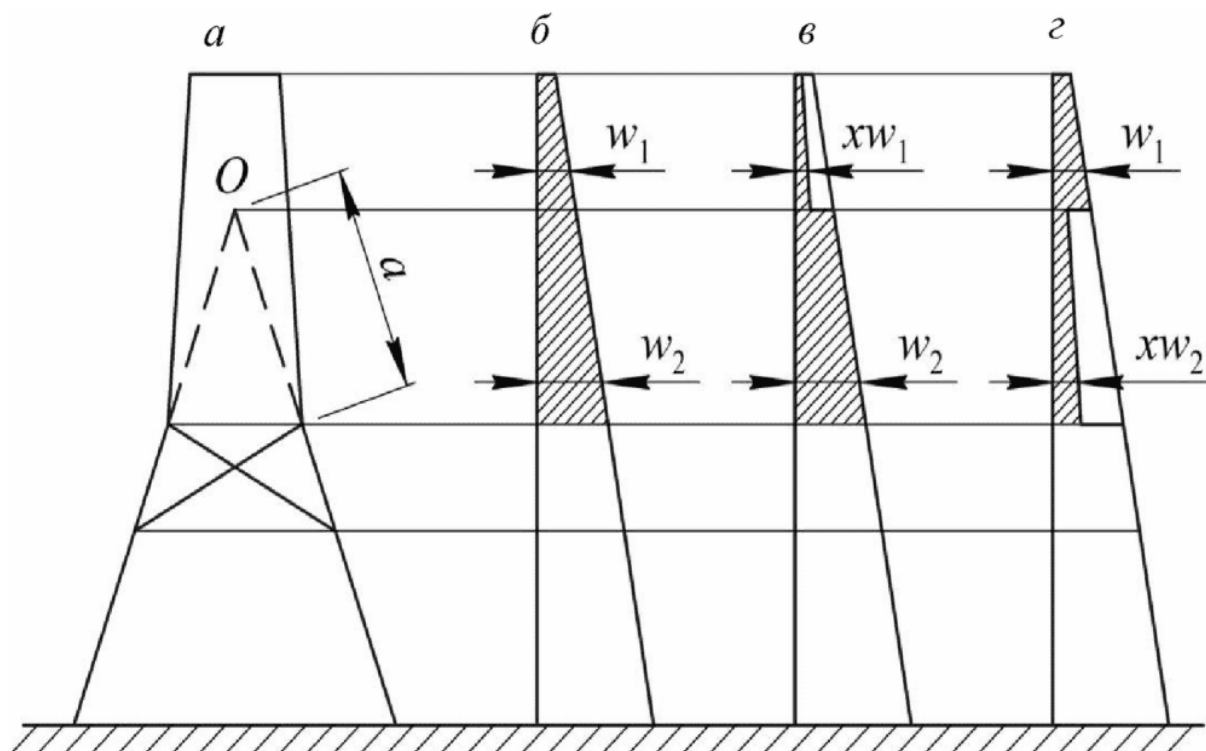
а - условная схема башни с точкой схода поясов О ; б - расчетная эпюра ветровой нагрузки на башню; в - эпюра ветровой нагрузки на башню с учетом уменьшения ветровой нагрузки на участке выше схода поясов; z - эпюра ветровой нагрузки на башню с учетом уменьшения ветровой нагрузки на участке ниже схода поясов
