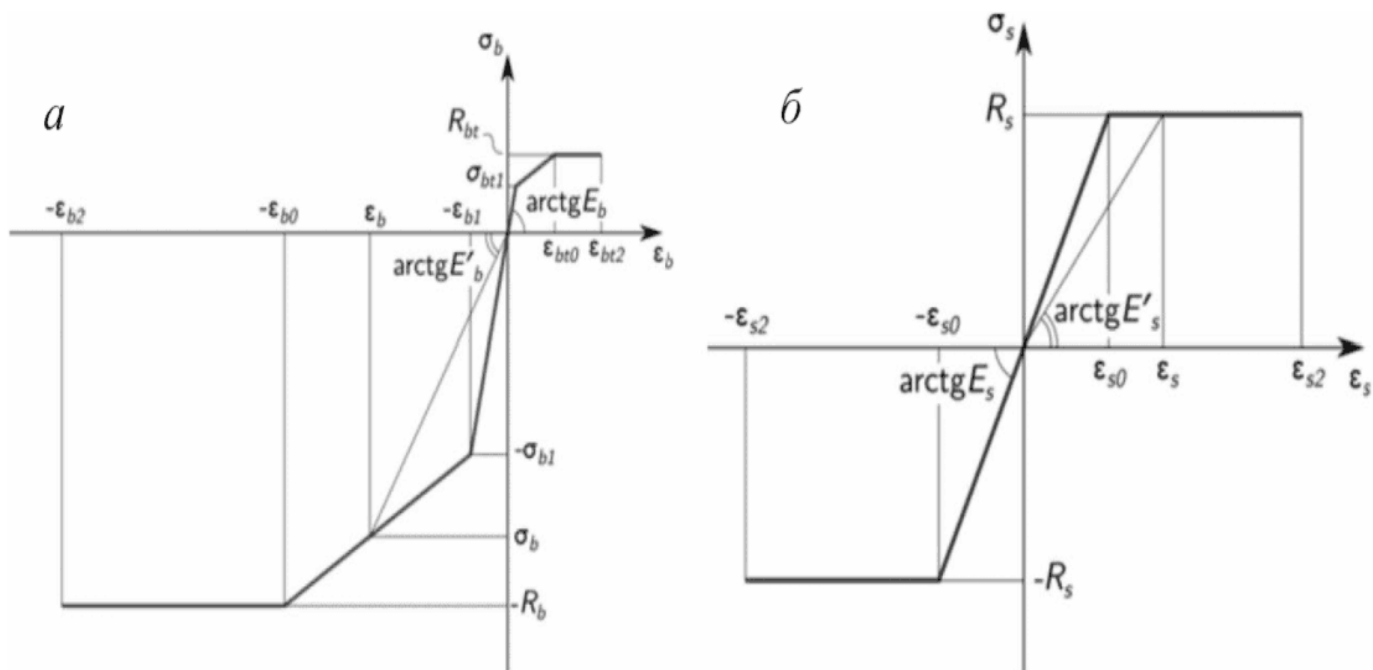
Рисунок Б.2 - Диаграммы деформирования бетона (а) и арматуры (б)
