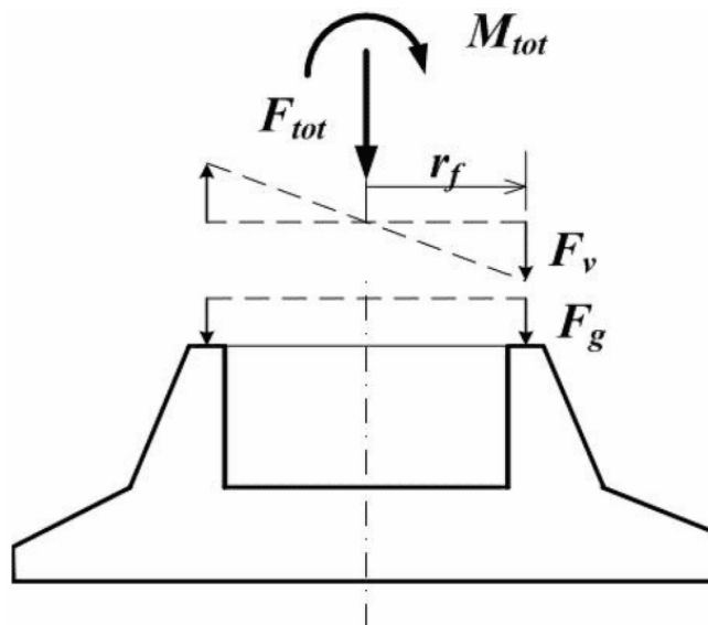
Рисунок 9.2 - Нагрузки от ствола трубы
