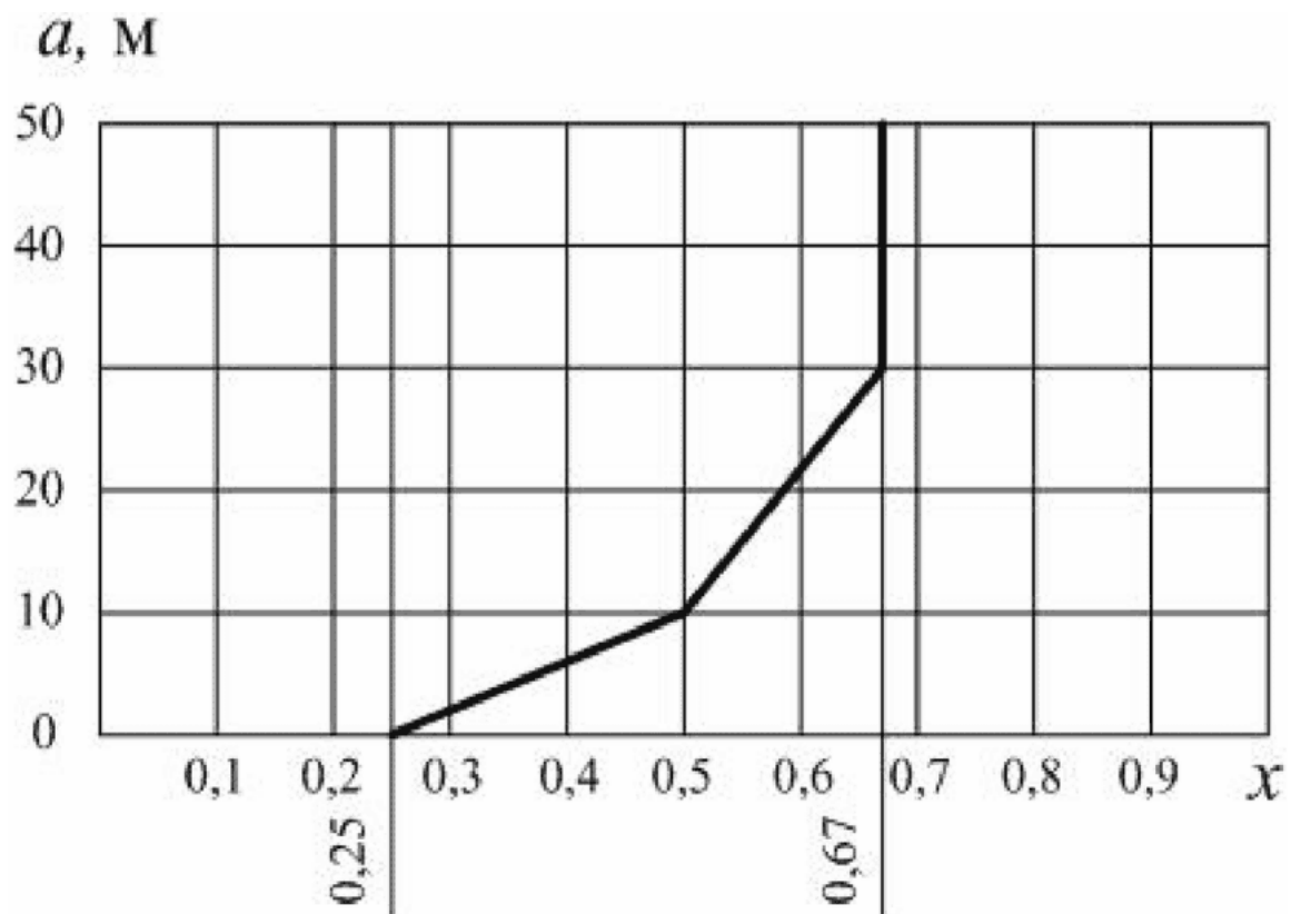
Рисунок А.2 - График для определения значения коэффициента x при зональном действии ветра
